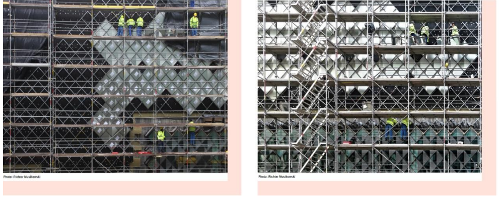
Şekil 17. İkinci aşamanın uygulanması ve diyağridler üzerine kasetlerin yerleşimi ( https://www.arup.com/news-and-events/modularization-meets-variability-futurium-showcases-curtain-walling-of-tomorrow )
